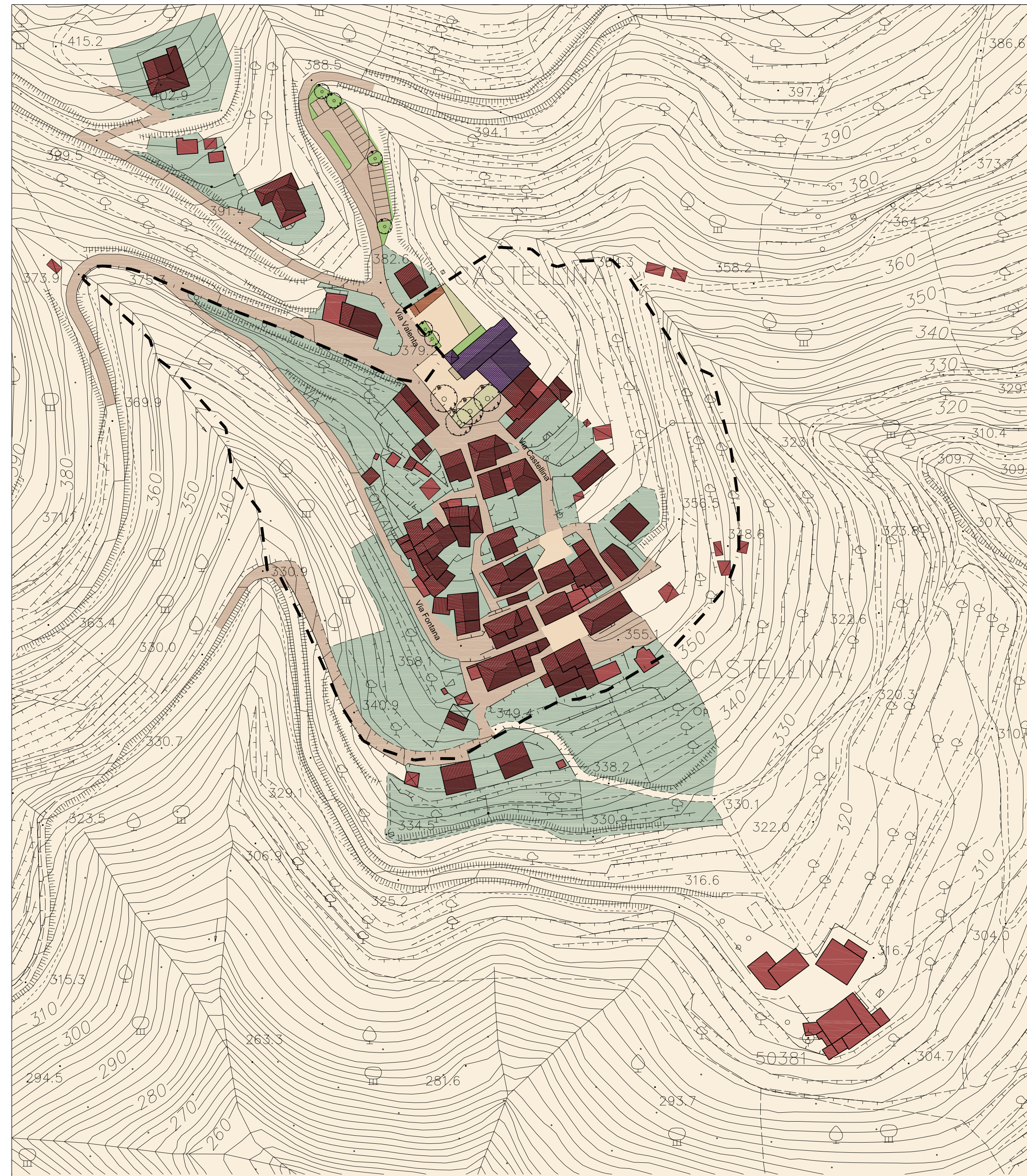
Planimetria scala 1:1000
