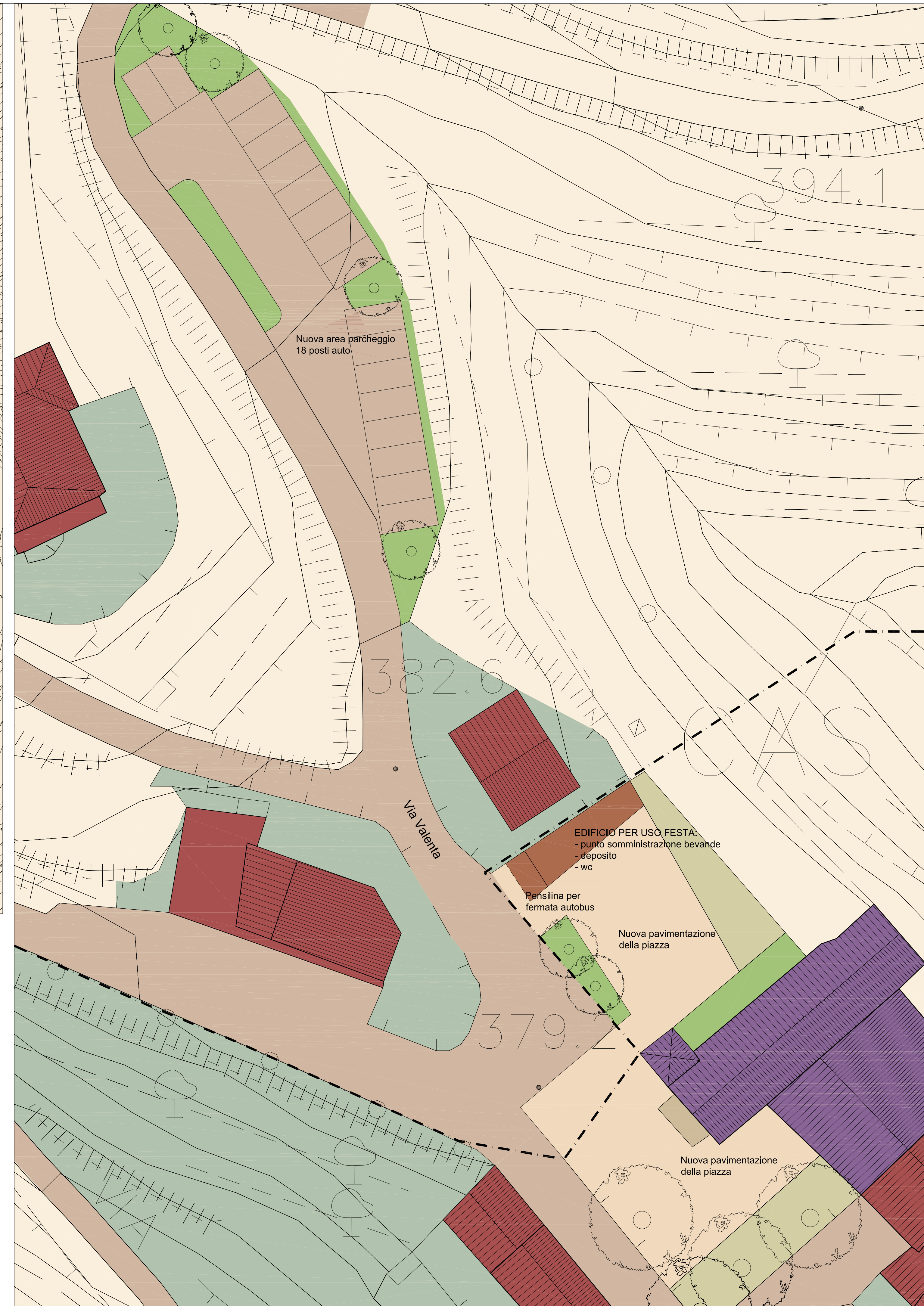
Planimetria scala 1:200
